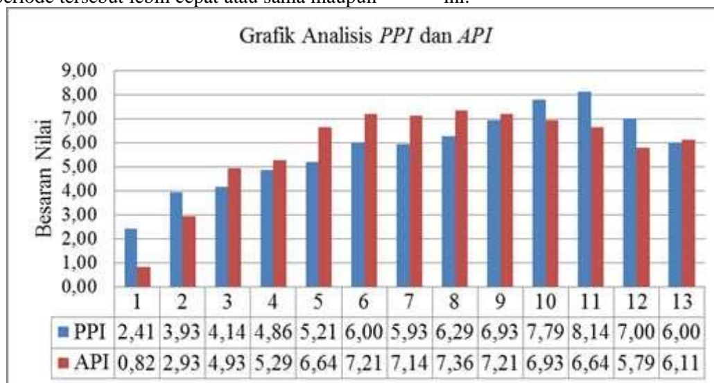
Gambar 2. Kinerja Waktu Proyek Per Periode pada Proyek Pembangunan Gedung Puskesmas Prambonwetan Kecamatan Rengel Tuban.
